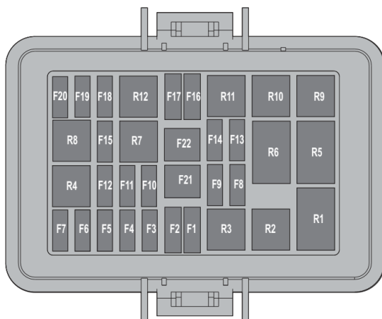
Schéma umístění pojistek
