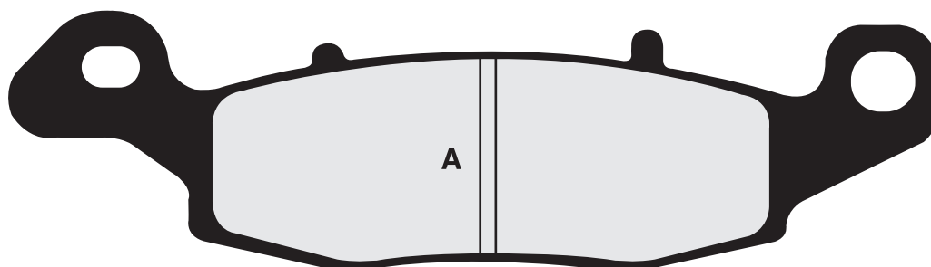
FRDB2750 • A. 133.50 x 36.80 x 8.40mm
