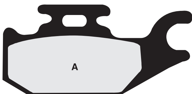
FRDB2400 • A. 82.08 x 40.85 x 9.46mm - B. 62.03 x 40.80 x 9.46mm
