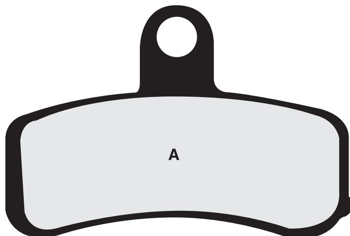
FRDB2168 • A. 90.60 x 62.10 x 8.10mm
