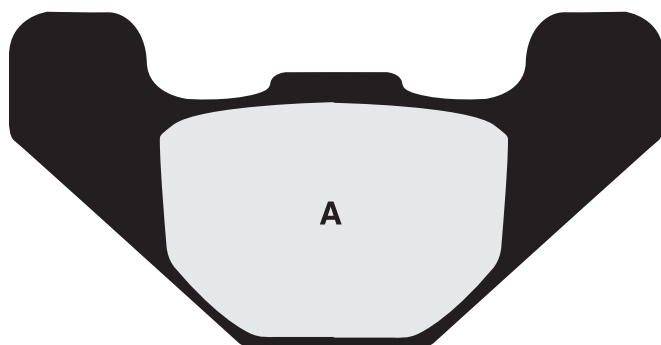
FRDB2159 • A. 85.12 x 42.70 x 7.40mm - B. 56 x 34.75 x 9.6mm
