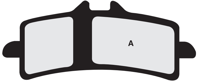
FRDB2154 • A. & B. 102.25 x 42.25 x 7.50mm
