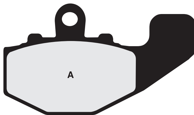
FRDB2042 • A. 90 x 51 x 8.50mm
